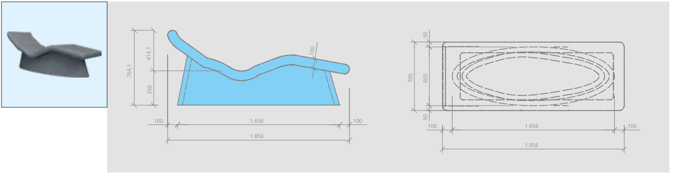
wedi Sanoasa® lounger 3
