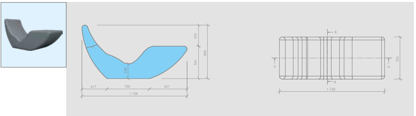
wedi Sanoasa® lounger 5
