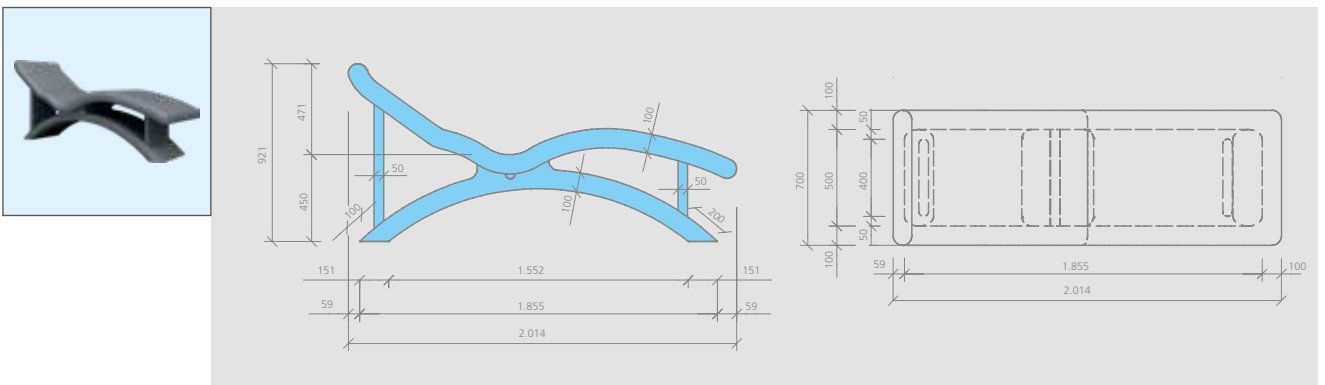
wedi Sanoasa® lounger 4
