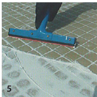
5 Levitä saumauslaasti (0-4 mm, Puk- kila Erikoissauma) kumisella sauma- lastalla.
