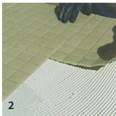
2 Aseta matot kiinnityslaastikerrok- seen nuolen osoittamaan suuntaan.
